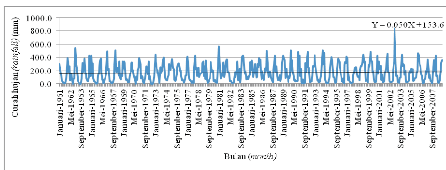
Gambar 4. Curah hujan bulanan periode tahun 1961-2008 Figure 4. Monthly rainfall pattern for 1961-2008 period
