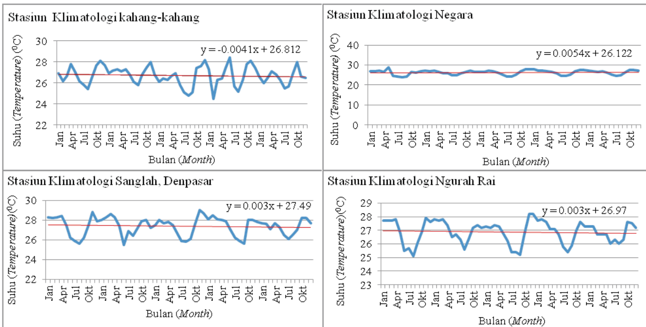
Gambar 8. Pola suhu bulanan-rata-rata dari tahun 2004-2008 Figure 8. Pattern of monthly average temperature for 2004-2008 period
