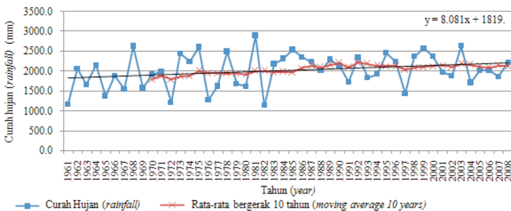
Gambar 5. Pola curah hujan tahunan di pulau Bali periode tahun 1961-2008 Figure 5. Annual rainfall pattern in Bali island for of 1961-2008 period
