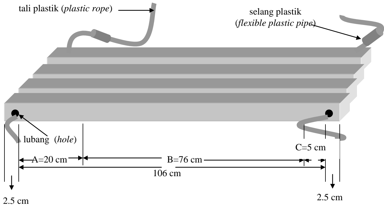
Gambar 1. Contoh uji yang dipasang di laut (A= contoh uji MCS; B= contoh uji lentur statik; C= contoh uji BJ, kerapatan dan kadar air).
