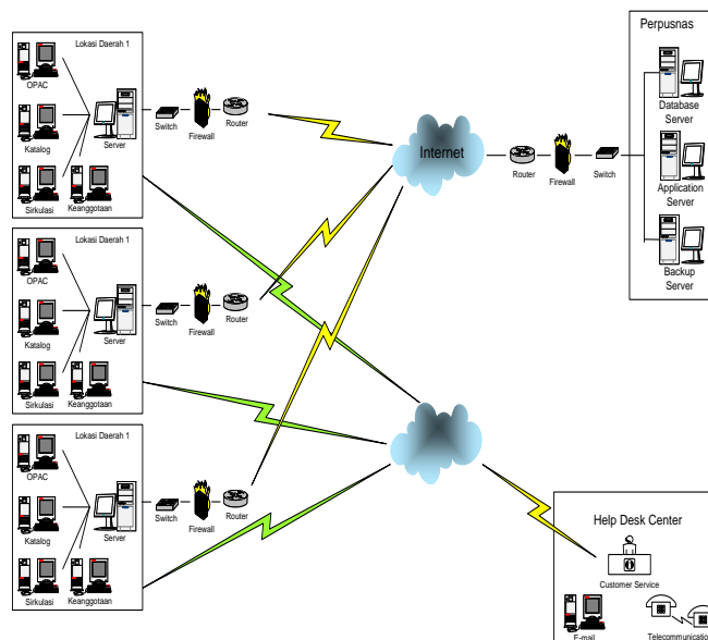
Bagan 1. Arsitektur Aplikasi Pangkalan Data Metadata Nasional - KIN dan BNI
